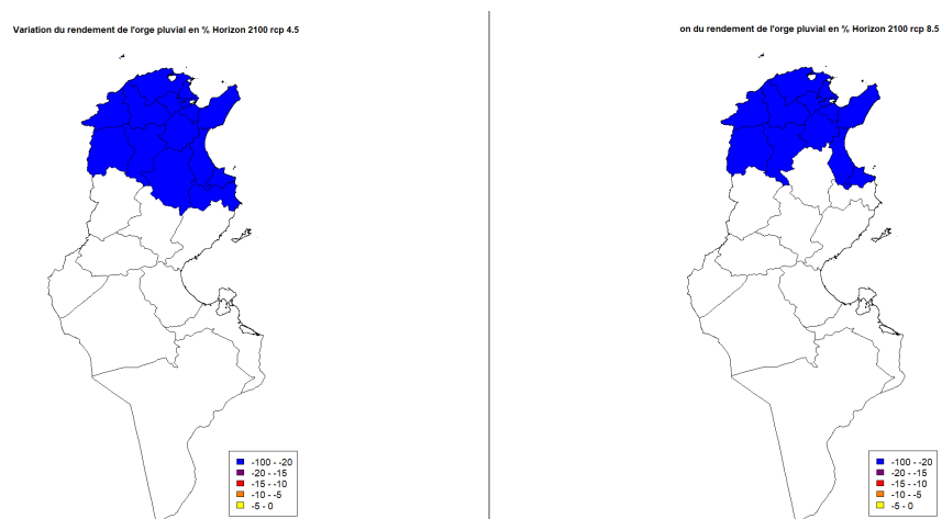
Figure 22 : Variation du rendement de l'orge pluvial horizon 2050 et 2100 / période de référence en %
