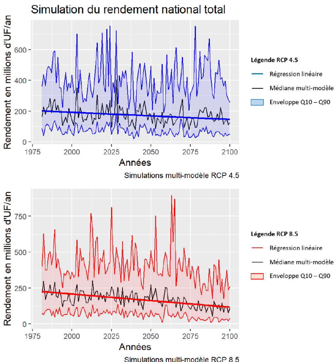
Figure 34 : Comparaison de la production fourragère des parcours de Tunisie pour les scénarios RCP4.5 et RCP8.5 en termes de médiane multimodèles avec Q10 et Q90
