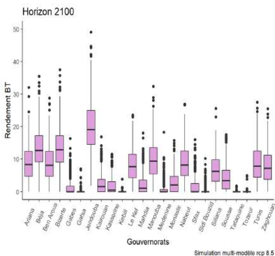
Figure 24 : Variation interannuelle et inter modèle des rendements du BLE TENDRE (qx/ha) par gouvernorat
