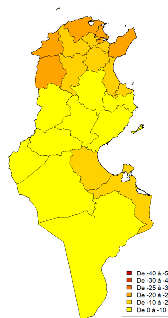
Variation du rendement des parcours (%) à l'horizon 2050 selon le RCP8.5
