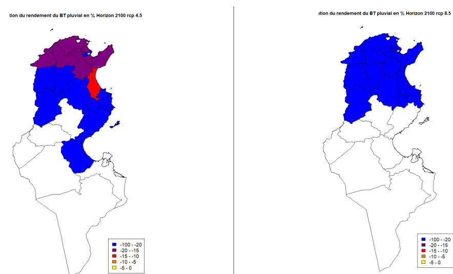
Figure 21 : Variation du rendement du blé tendre pluvial horizon 2050 et 2100 / période de référence en %
