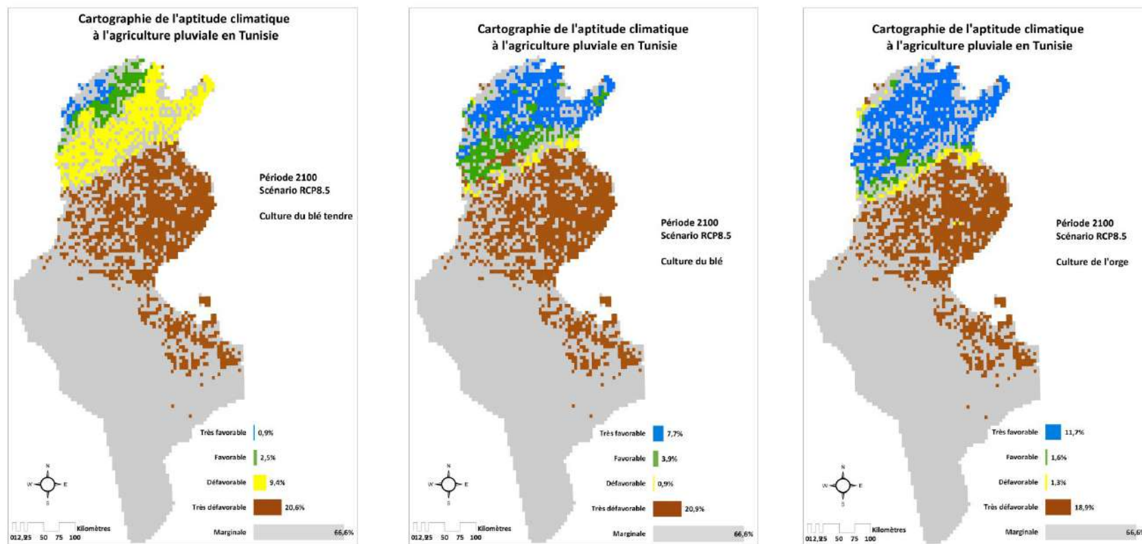
Figure 26: Cartographie de l'aptitude climatique à la culture des céréales à l'horizon 2100 pour le scénario RCP8.5.
