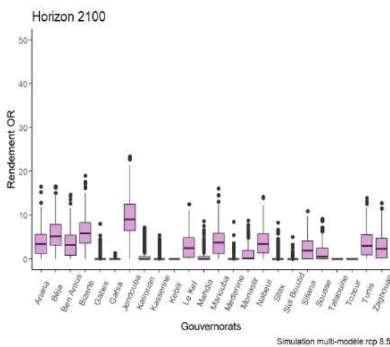
Figure 25 : Variation interannuelle et inter modèle des rendements de l'ORGE (qx/ha) par gouvernorat
