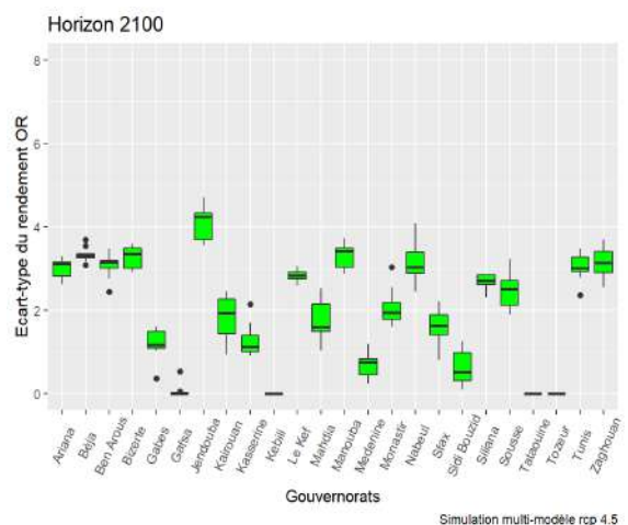
Figure 19 : Variation interannuelle et inter modèle des écarts type des rendements de l'orge
