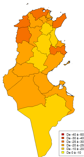
Variation du rendement des parcours (%) à l'horizon 2100 selon le RCP4.5
