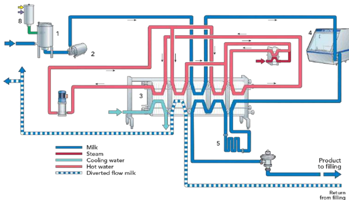
Figure 3. Procédé UHT par chauffage indirect dans un échangeur de chaleur à plaques
