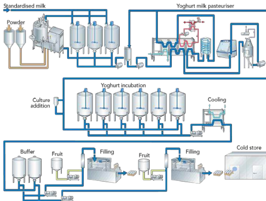
Figure.9 Ligne de production du yaourt brassé
