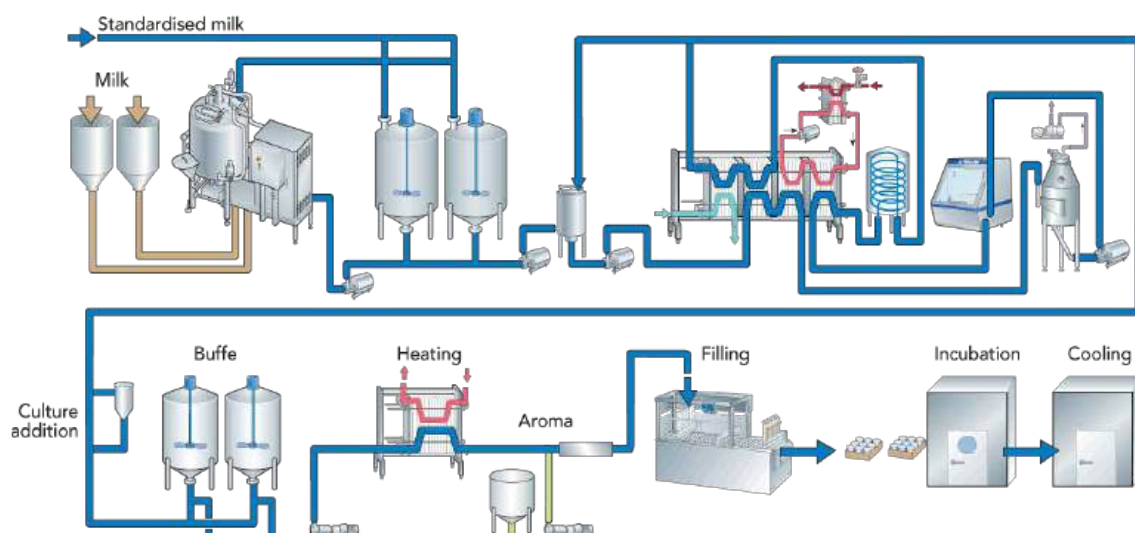
Figure.8 Ligne de production du yaourt ferme
