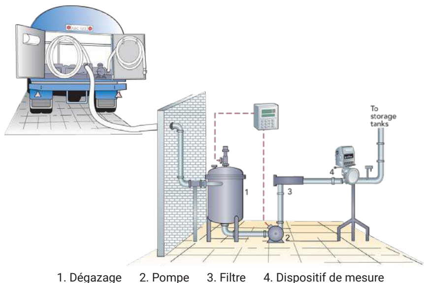
Figure.5 Réception du lait à la laiterie: dégazage et mesure volumétrique
