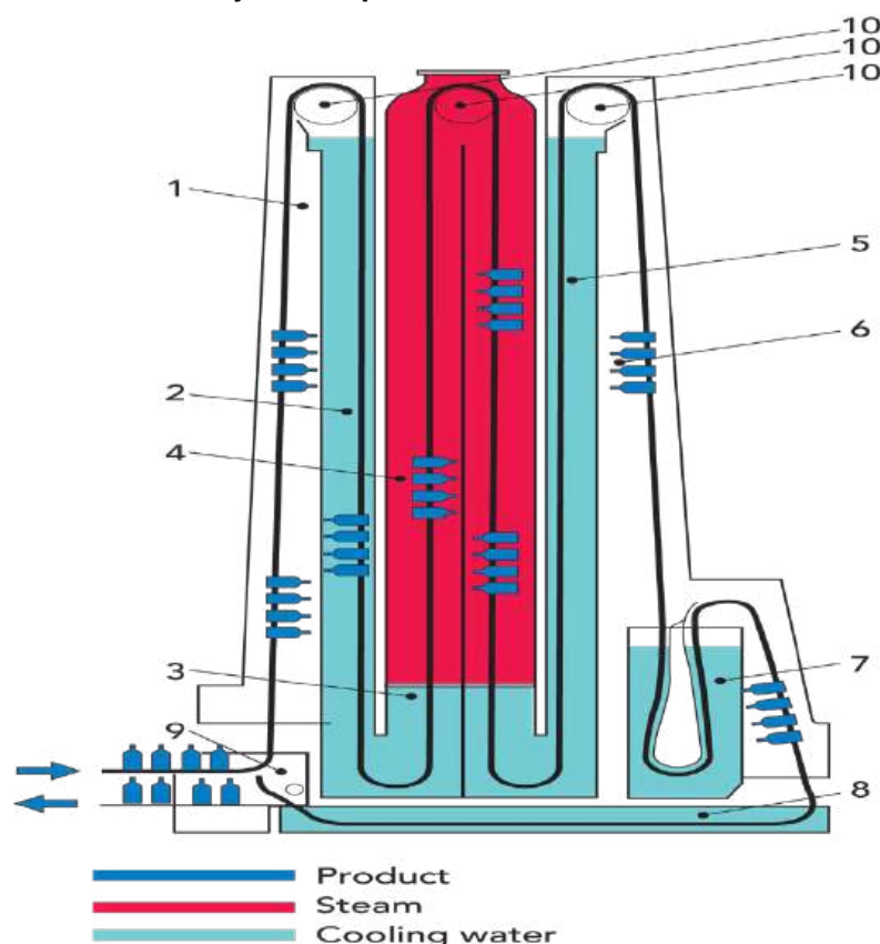
Figure.4 Stérilisateur vertical hydrostatique
