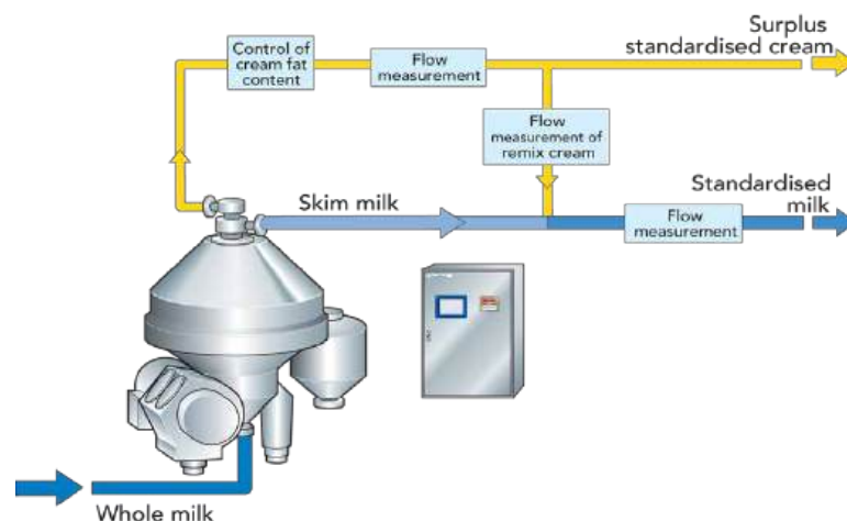
Figure.7 Système de standardisation automatique du lait en matière grasse
