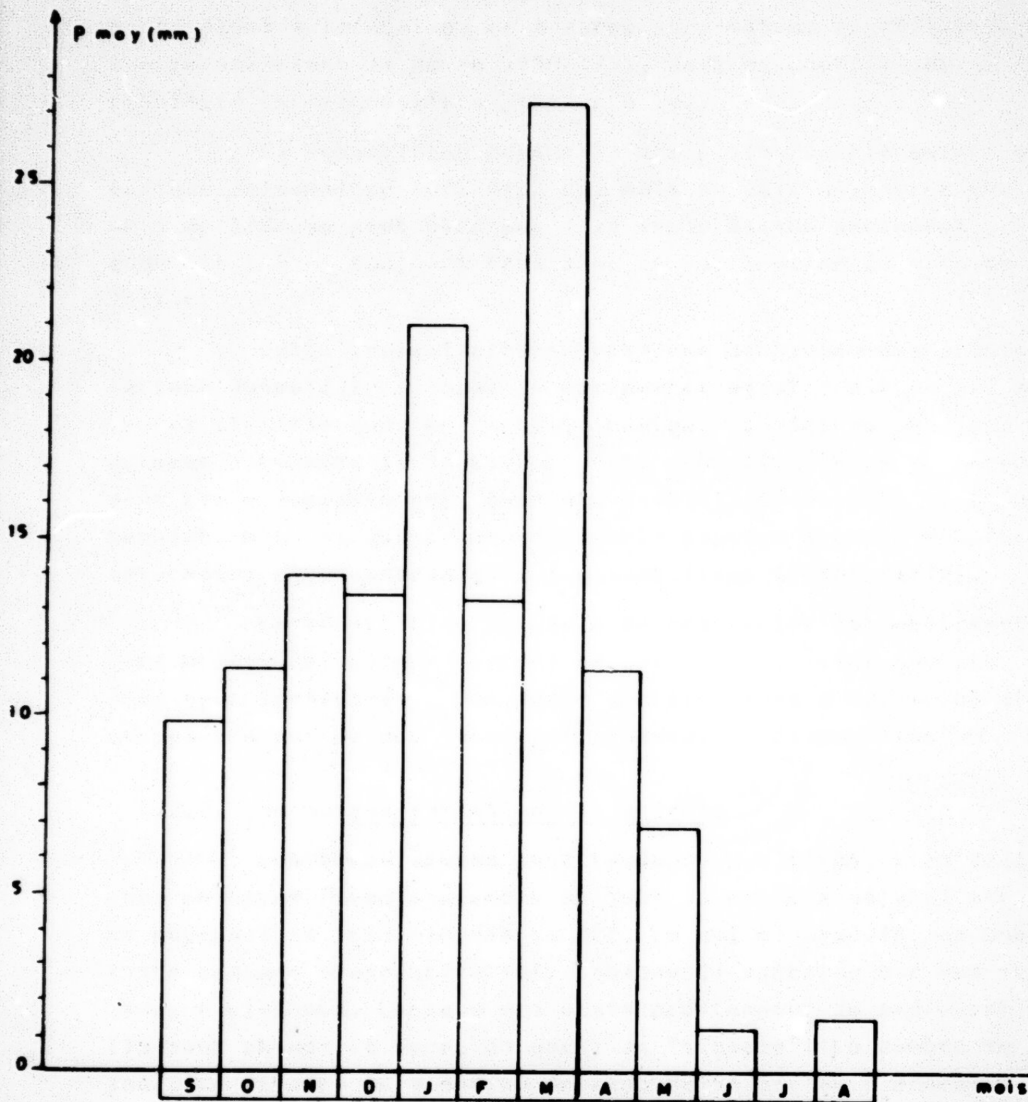
Fig. n° 2 PRECIPITATION MOYENNES MENSUELLES A TATAOUMNE
